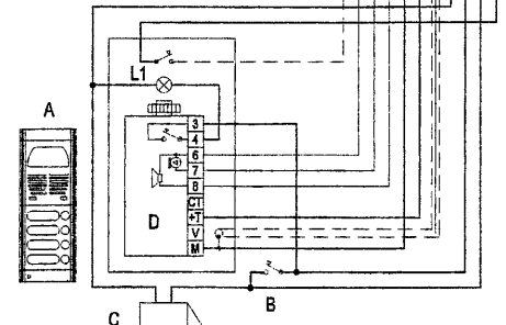
DIAGRAM N° vc3242
