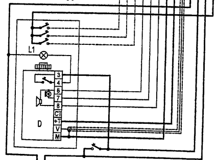
DIAGRAM N° vc4306
